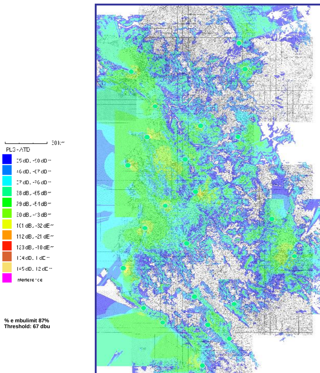
Fig.6 Mbulimi me sinjal analog tokësor në bandën UHF, realizuar nga TVSH
