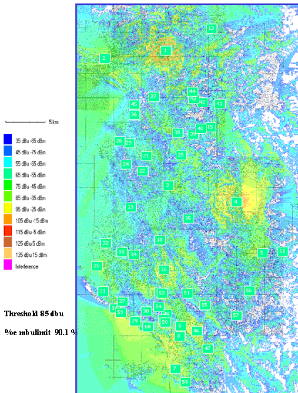
Fig. 5 Mbulimi me sinjal analog tokësor në bandën VHF, i realizuar nga TVSH
