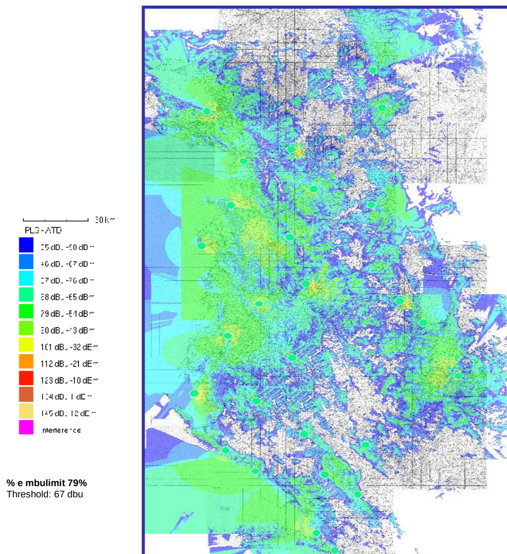
Fig. Mbulimi me sinjal analog tokësor në bandën UHF, realizuar nga Top Channel
