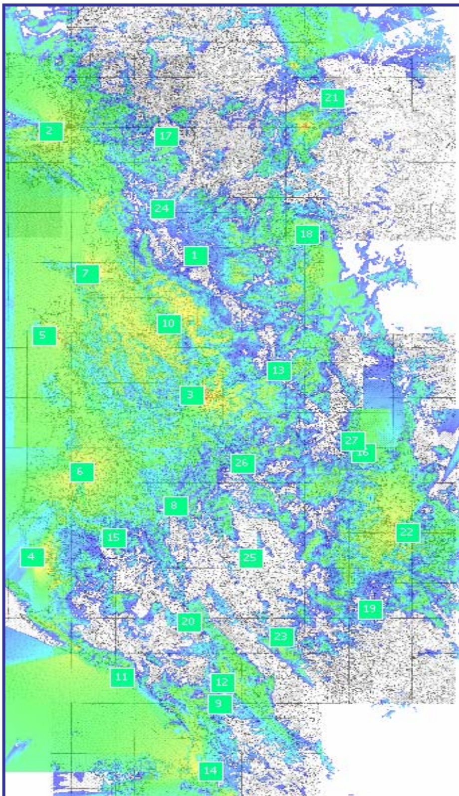
Fig.10 Mbulimi me sinjal analog tokësor i TV TOP CHANNEL në fund të vitit 2011
